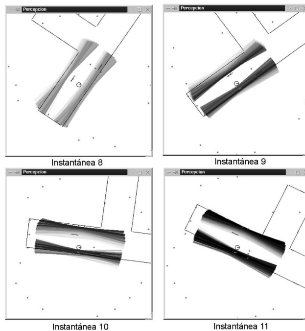
Figura 6: Seguimiento del pasillo moviéndose el robot en el entorno 1. El obstáculo puede verse como un segmento recto paralelo al pasillo.
