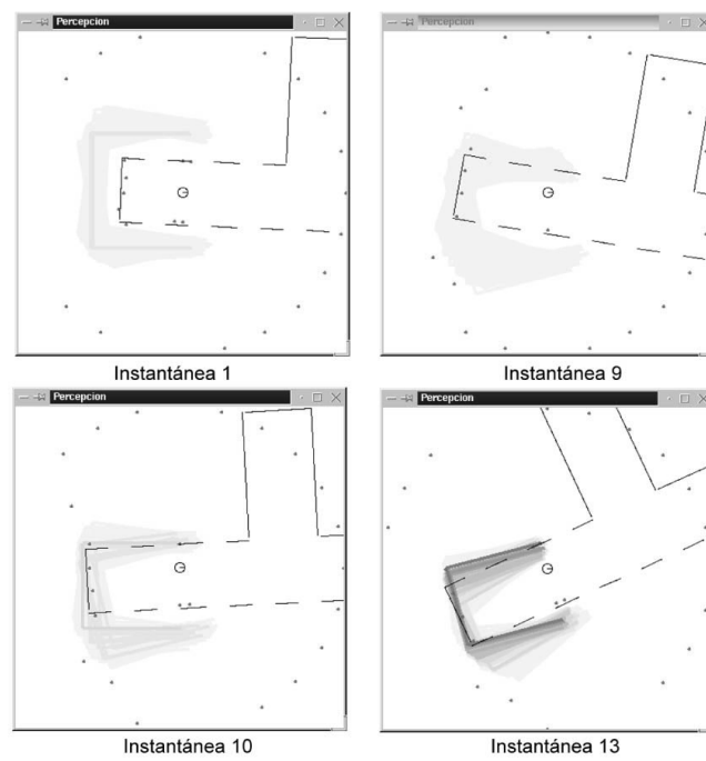
Figura 7: Seguimiento de finales de pasillo moviéndose el robot en el entorno 2.
